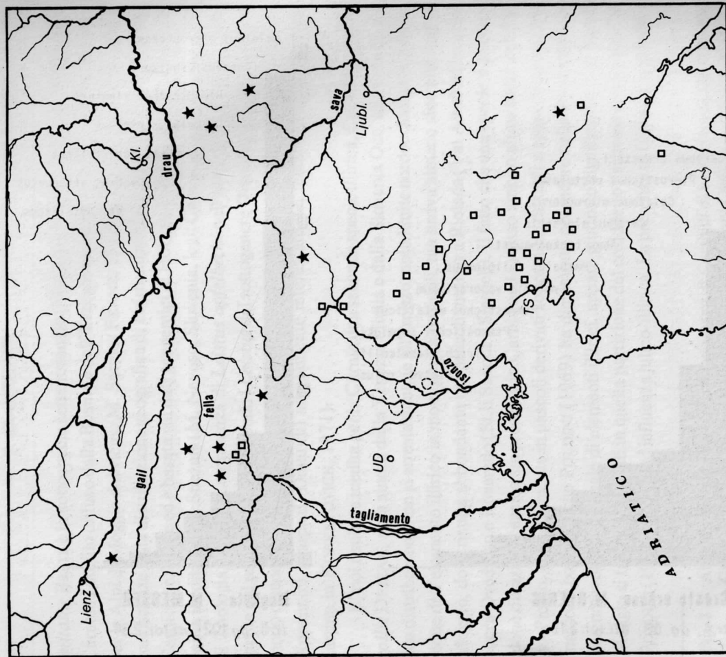
Fig. 4 - Penetrazioni illiriche nelle Alpi d'Incaroio. Stelle: distribuzione geografica di Leistus imitator (= L. apfelbecki ssp. imitator ) secondo HÖLZEL (1958), integrata con dati inediti di CASSOLA per il M. Snežnik (M. Nevoso, Slovenia, YU, 14/VIII/1973) coll. VIGNA, Ist. Zoologia, Roma. La specie in toto è diffusa dalla Bosnia alle Alpi Carniche. Quadri: Calathus glabricollis , geonemia delle sue popolazioni più settentrionali basata su MÜLLER (1926) e nostre raccolte. Le Alpi di Moggio rappresentano, allo stato attuale di approfondimento delle ricerche, il limite nord-occidentale di questa specie praticola montana dinarica. Illyrian penetrations in the Carnic Alps around Moggio Udinese. Stars: northern part of the area of Leistus imitator (= Leistus apfelbecki ssp. imitator ), localities by HÖLZEL (1958) and F. Cassola, unpublished. The whole of area ranges from Carnic Alps to Bosnia, Yugoslavia. Squares: Calathus glabricollis , northern part of the area by MÜLLER (1926) and author's catches. This montane meadow-dwelling beetle reaches on the Zuc del Boor (study area) the northwestern limit of its area.
