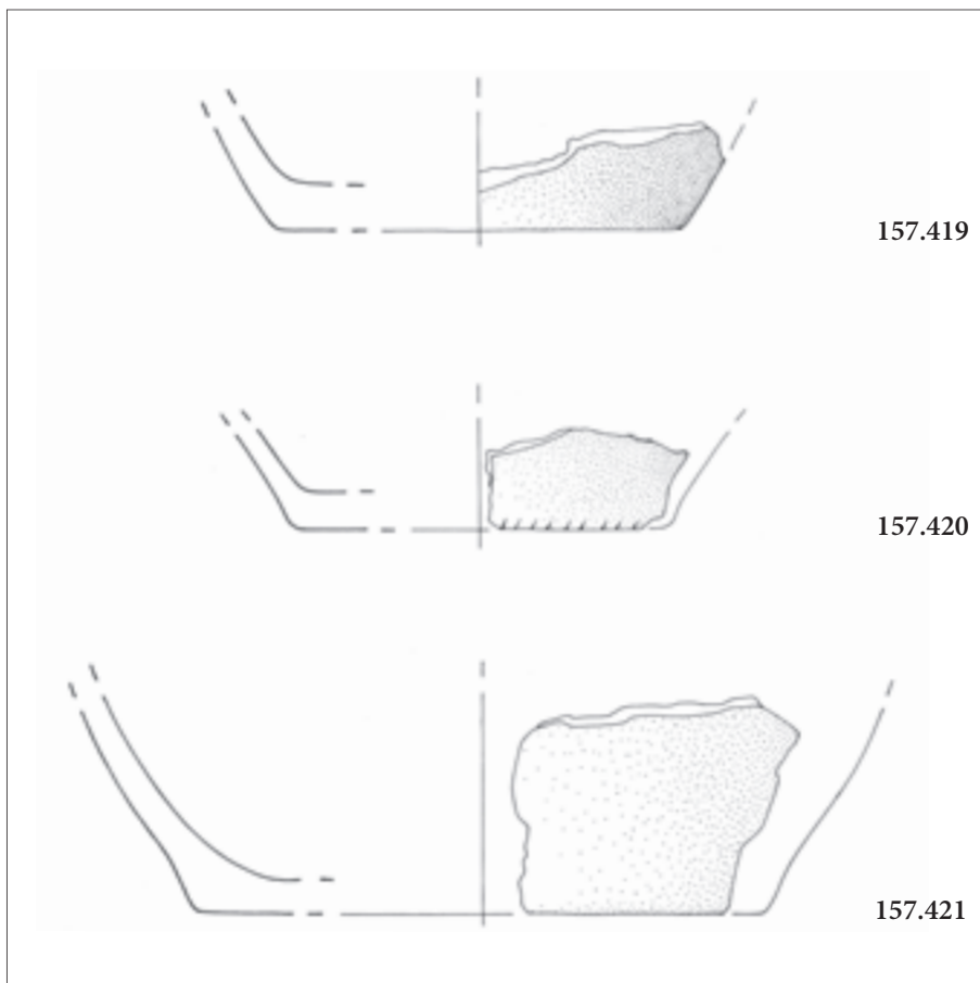
Fig. 5 - Fondi (dis. G. Merlatti; scala 2:3). - Bases (drawings by G. Merlatti; 2:3).
